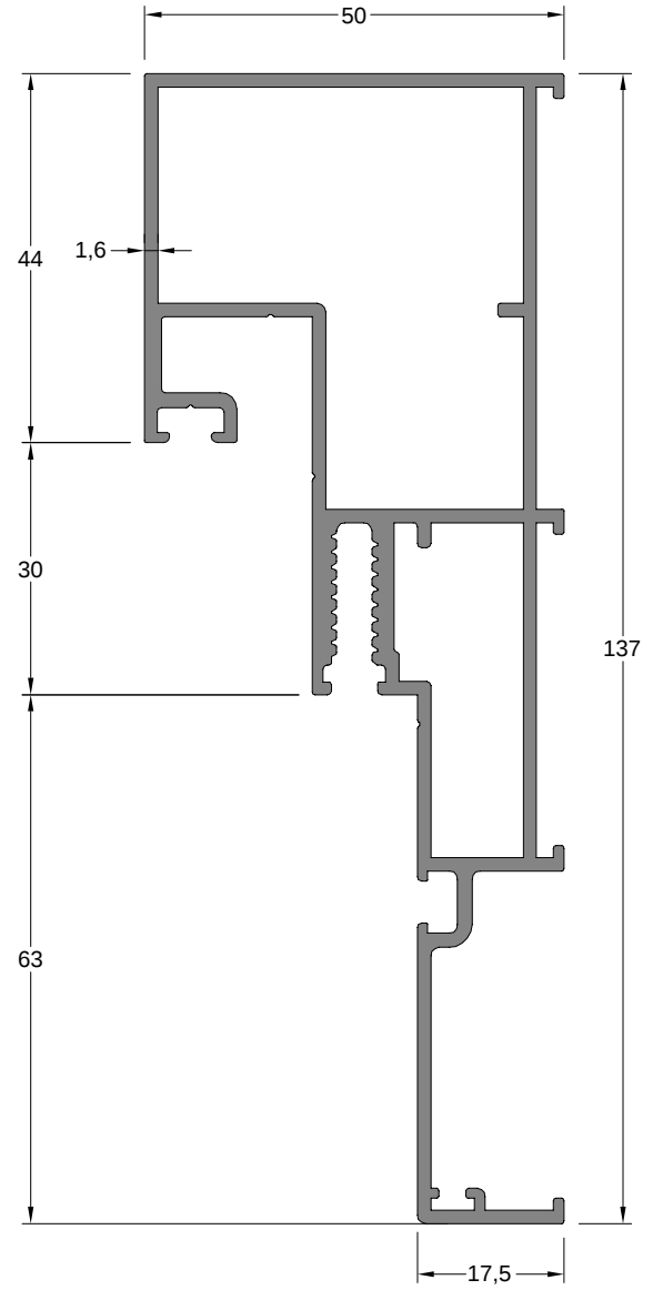
Tırnaklı sistem duvar bitiş profili Finish Profile
