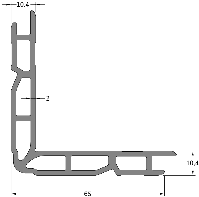
Köşe Takoz Profili Corner wedge profile
