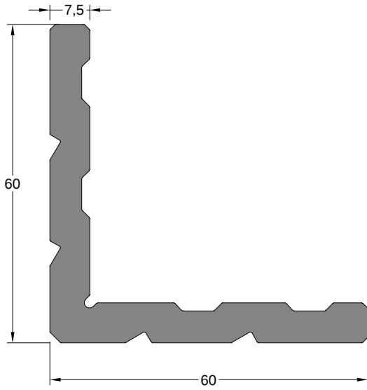
Köşe Takoz Profili Corner wedge profile
