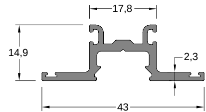
Baskı profili Frame Profile
