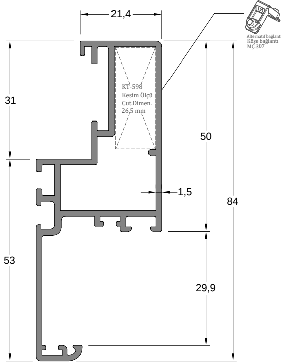
Tırnaklı Kaset Profili Casedde Profile
