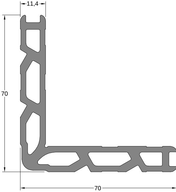
Köşe Takoz Profili Corner wedge profile
