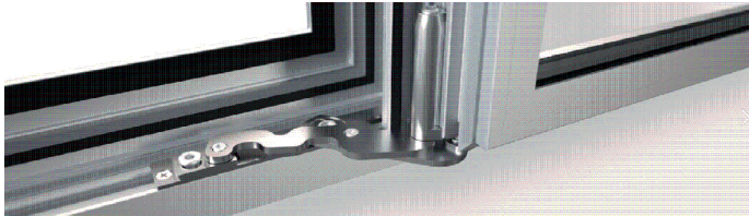
giesse gizli menteşe çift açılım seti 100 kg giesse hidden hinge tilt & turn mechanism 100 kg
