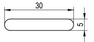
TAHLİYE DELİĞİNİN ÖLÇÜLERİ DRAINAGE HOLE DIMENSIONS
