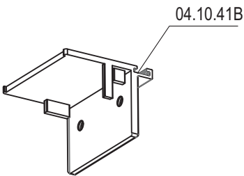
* PVC KAPAK (ÜST) PVC CAP (UPPER) Malzeme / Material : PVC (RMS45 V 04 - RMS45 V 05 için / for RMS45 V 04 - RMS45 V 05)
