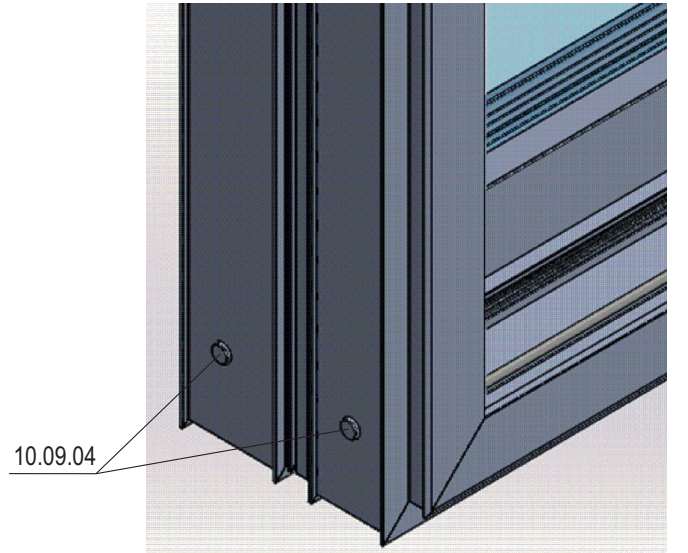
Köşe Detayı 3d Görseli
